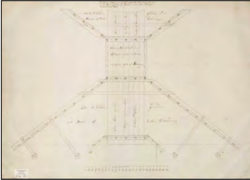
De bemaling van de molenviergang kruiste de molenwetering van de Zuideinderpolder. Daarvoor moest een duiker worden aangelegd, waardoor de boezem tussen de molens 2 en 3 (toen aangeduid als de molens 1 en 2) onder de dwarswetering door ging. (collectie hoogheemraadschap van Rijnland)
