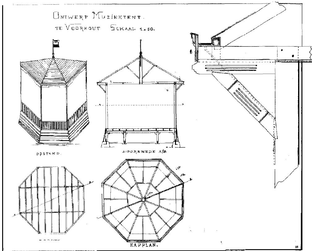
Bouwkundige tekeningen van de muziektent. Reconstructietekening naar een slechte negatieve blauwdruk, door Emiel van der Hoeven, 1995.
